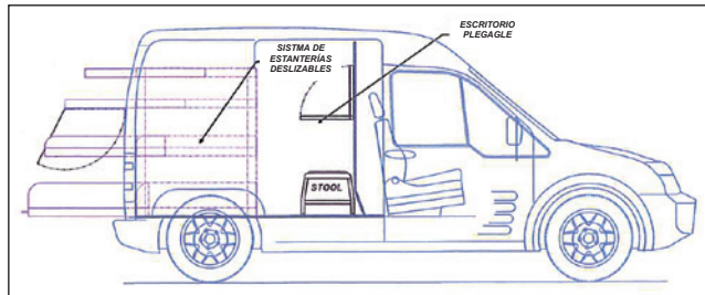
Vista interior del lado de la calle del equipo ECV100/TC
